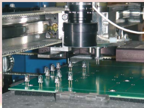
LED-Bestückungsautomat
